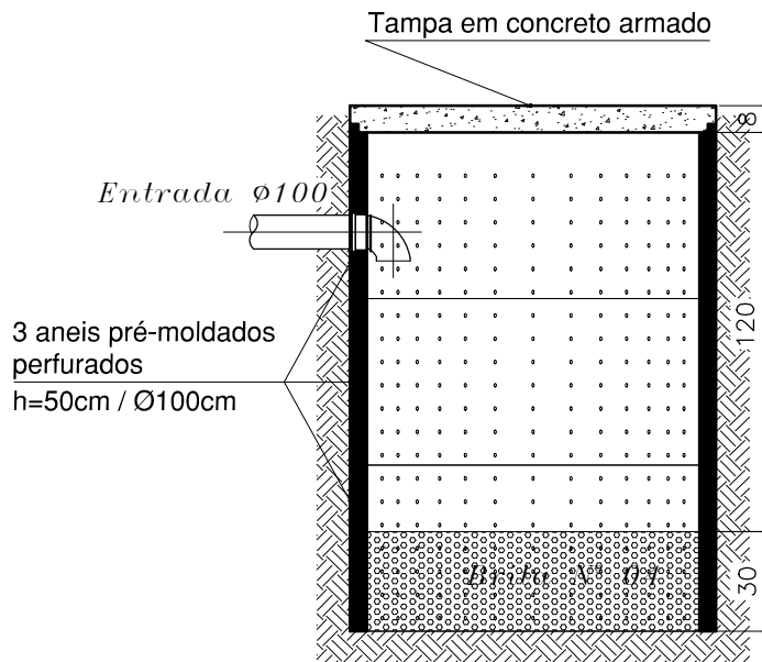
1 DETALHE SUMIDOURO
